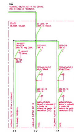
ESQUEMA UNIFILAR QUADRE ALIMENTACIÓ MÀQUINES SENSE ESCALA
