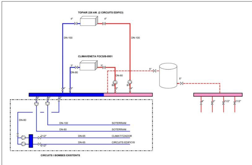
ESQUEMA IMPLANTACIÓ DE NOUS EQUIPS I CONNEXIÓ A INSTAL·LACIÓ EXISTENT SENSE ESCALA
